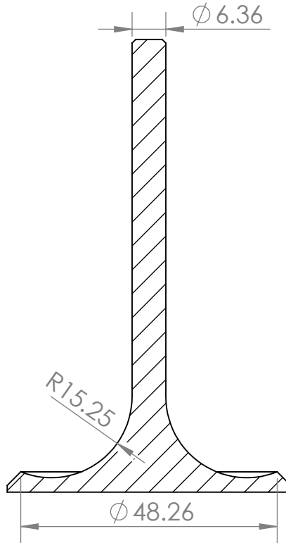
SECTION A-A SCALE 1 : 1
